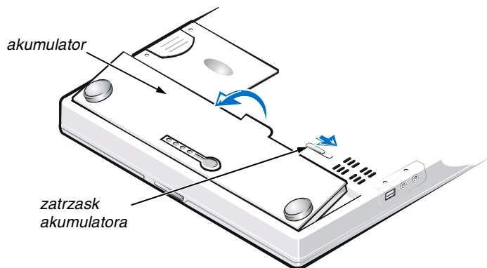
Rysunek 7-3. Wyjmowanie akumulatora
