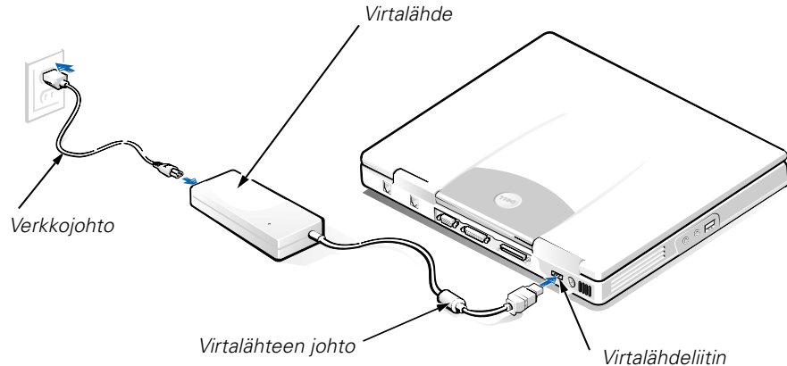
Kuva 4-1. Virtalähteen kytkeminen
