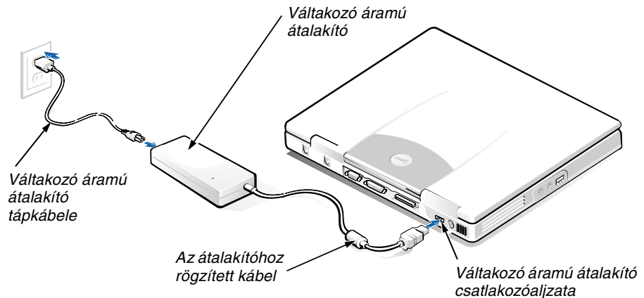
5.1. ábra. A váltakozó áramú átalakító csatlakoztatása
